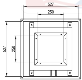
MẶT TRÊN
