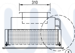
MẶT CẮT
