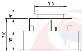
MẶT TRƯỚC
