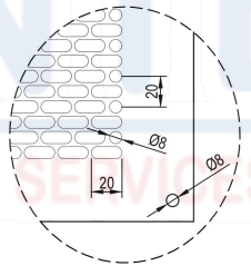
CHI TIẾT 2
