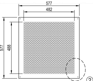
MẶT DƯỚI
